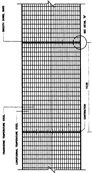
แบบแปลนของงานโยธา
