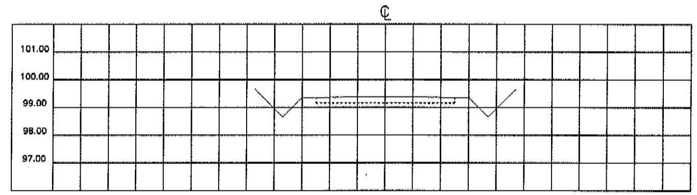
STA 1+100
