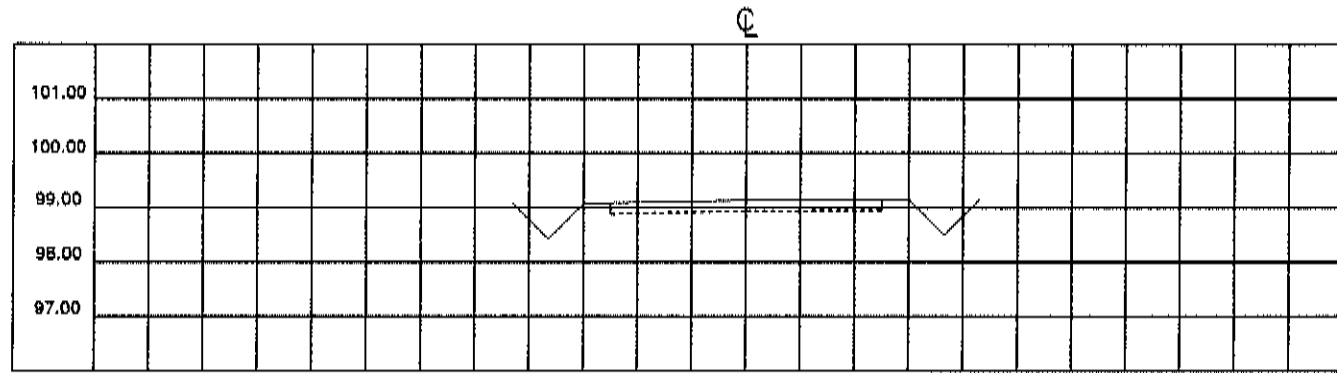
STA 1+450
