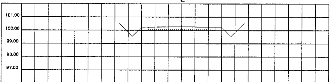
STA 0+000
